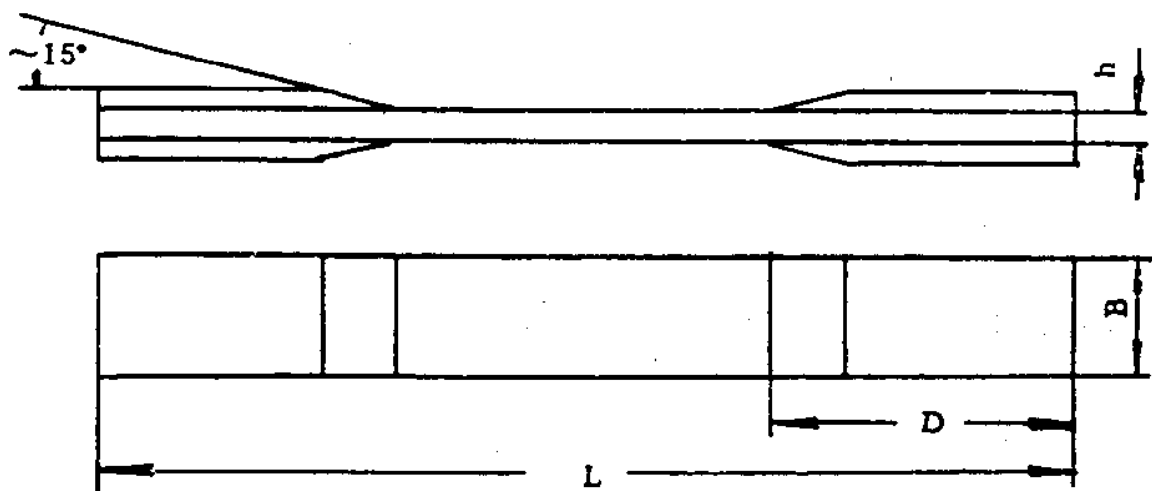
图 2 试样
