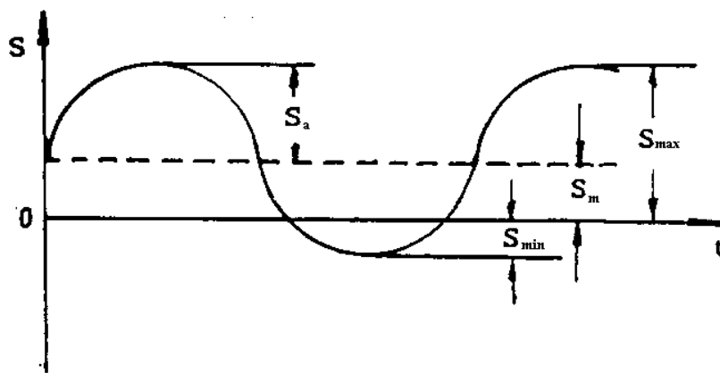
图 1 疲劳试验参数
