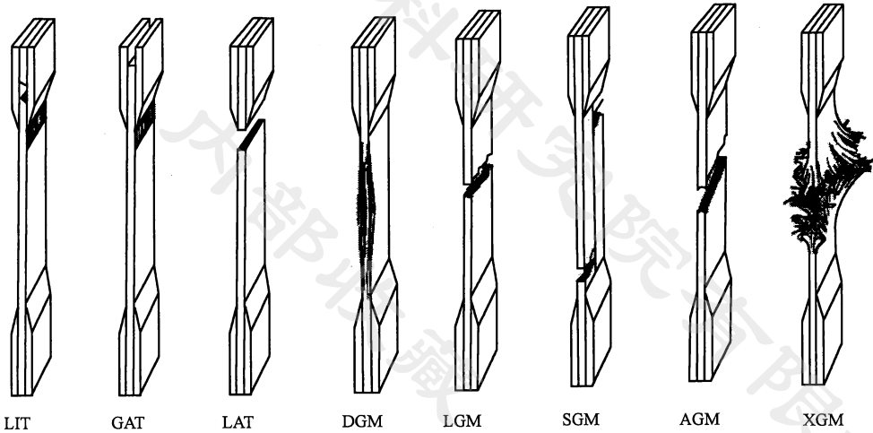
图 4 拉伸试验的典型失效模式示意图
