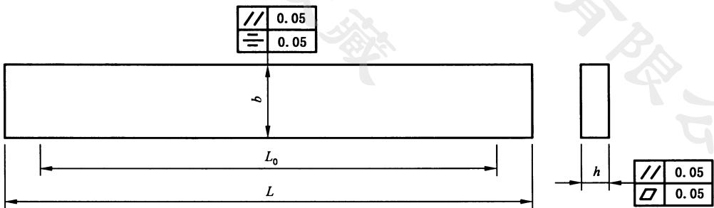
图 8 弯曲试样型式
